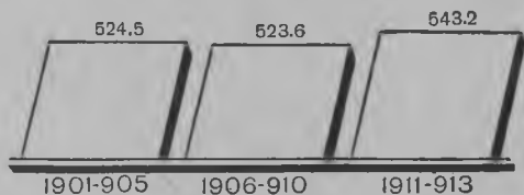
Средний ежегодный вывоз хлеба из России в 1901—1913 годах (в млн. пуд.).
